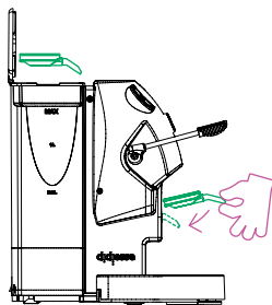
Fig. 9-B - prelevare l'erogatore per l'acqua calda e inserirlo al posto del portacialda precedentemente rimosso
