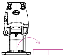
Fig. 9-C - rimuovere la vaschetta di raccolta
