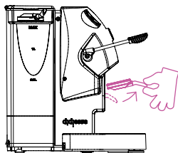
Fig. 10-B - sollevare ed estrarre il portacialda per l'erogazione del caffè
