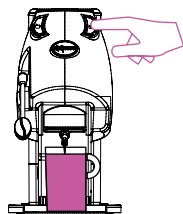
Fig. 9-F - raggiunta la temperatura di esercizio, il pulsante emanerà luce fissa. Premere il pulsante per erogare la quantità di acqua calda desiderata e ripremere per interrompere l'erogazione
